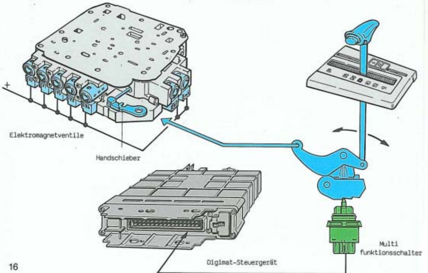
Schieberkasten
